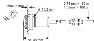
Capteur de luminosité encastrable
